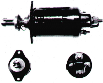
REF.ORIGINAL FYRECO CED 2052 AMT-2052 PARA ARRANQUES: D11E2124,38. Camiones Ebro.
