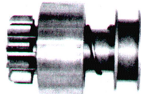
REF.ORIGINAL FYRECO 6320004. PIMT-004 PARA ARRANQUES: Tractores Ebro. L: 77 NºDIENTES: 10 NºESTRIAS INT: 6 Helicoi.
