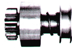
REF.ORIGINAL FYRECO 6320007. PIMT-007 PARA ARRANQUES: D11E2124.Tractores Ebro. L: 87 NºDIENTES: 10 NºESTRIAS INT: 6 Helicoi.
