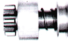
REF.ORIGINAL FYRECO 6320006. PIMT-006 PARA ARRANQUES: D11E2138.Camiones Ebro. L: 87 NºDIENTES: 11 NºESTRIAS INT: 6 Helicoi.
