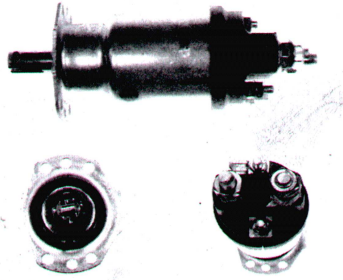
REF.ORIGINAL FYRECO CED 2141 AMT-2141 PARA ARRANQUES: D11E2136,78, 2001,8.Camiones Ebro.
